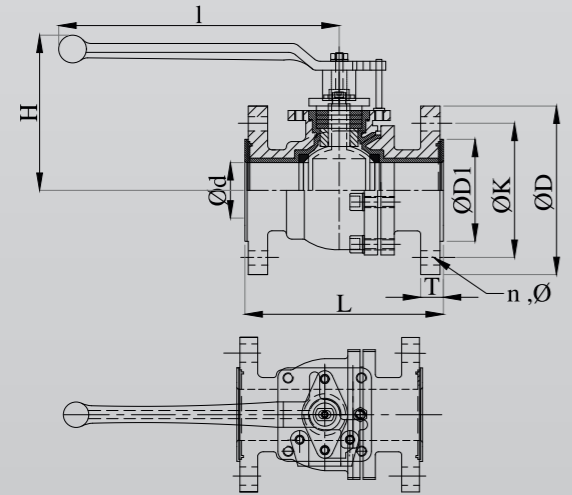
DIMENSIONS
