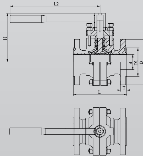
DIMENSIONS
